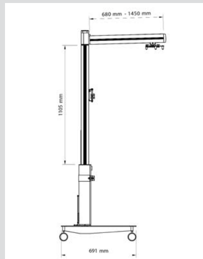
Vista lateral
